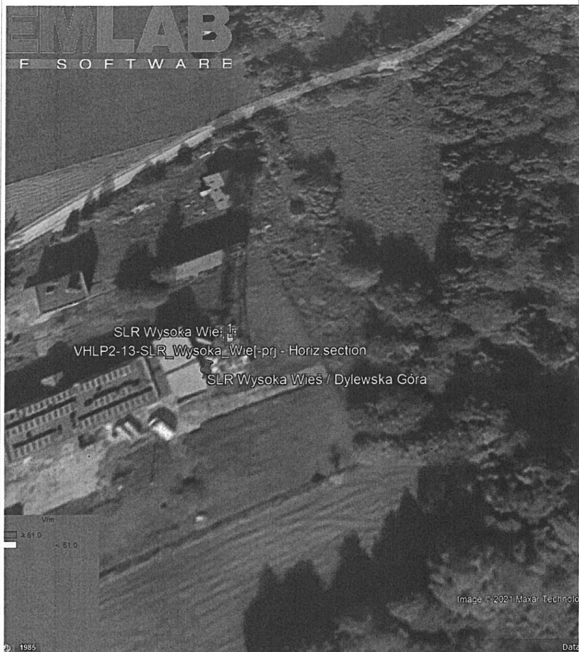
Rys. 2. Rzut poziomy rozkładu pola elektromagnetycznego anteny nowo projektowanej linii radiowej w otoczeniu SLR Wysoka Wieś/Dylewska Góra przewidzianej do zainstalowania na wysokości 35 m nad poziomem terenu.
